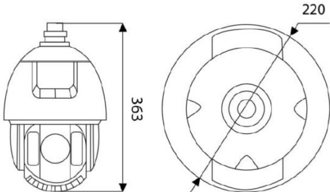
Abmessungen
