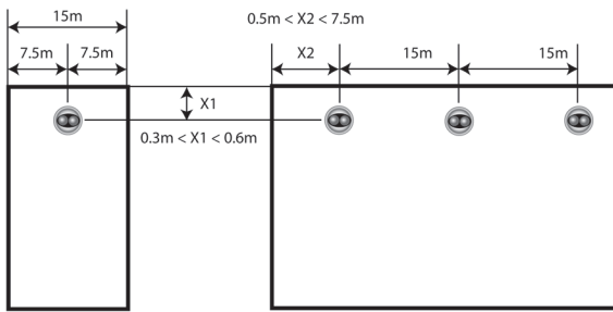
Flachdeckenmontage
