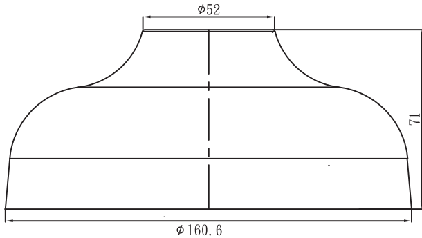
NDA-4020-PIP Hängeadapterplatte Abmessungen in mm
