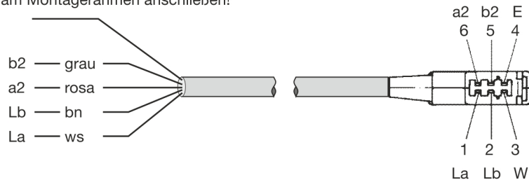
TAE - Anschlusskabel 5polig
